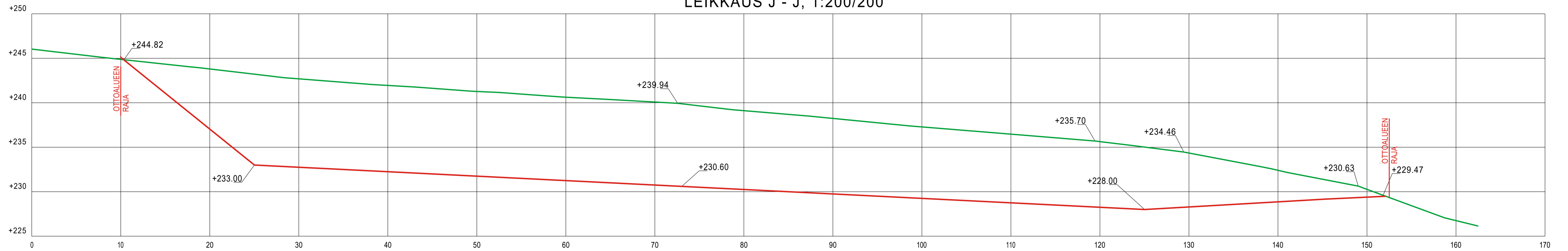
LEIKKAUS J - J, 1:200/200
