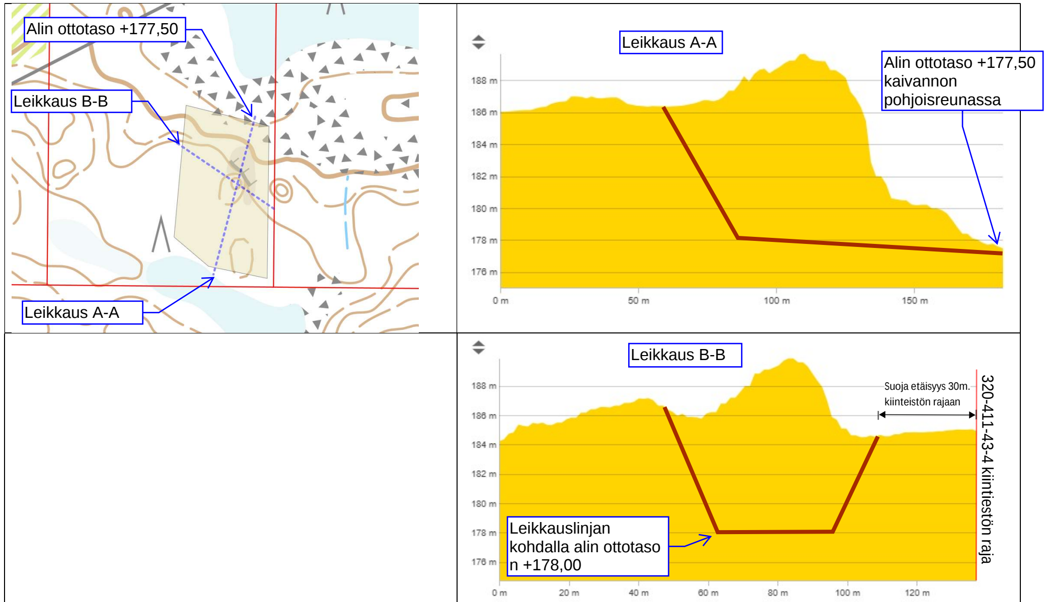
Liite 4, leikkauskuvat (täydennys ottorajan suoja-alueesta naapurikiinteistöön)
